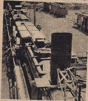
EEN ELECTRICHE CENTRALE OP WIELEN. Uit 8 wagons bestaande "treinen" worden door de Amerikanen naar Europa gebracht om verwoeste steden onmiddellijk van electrischen stroom te kunnen voorzien. Het vermogen van iedere centrale is 5000 K.W.
